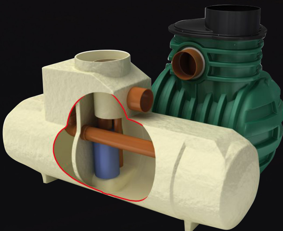
BYPASS-SEPARATOR NSBP-SERIEN
